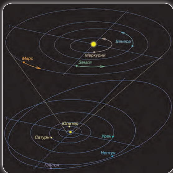
Положения планет на орбитах в июле 2014 г.
