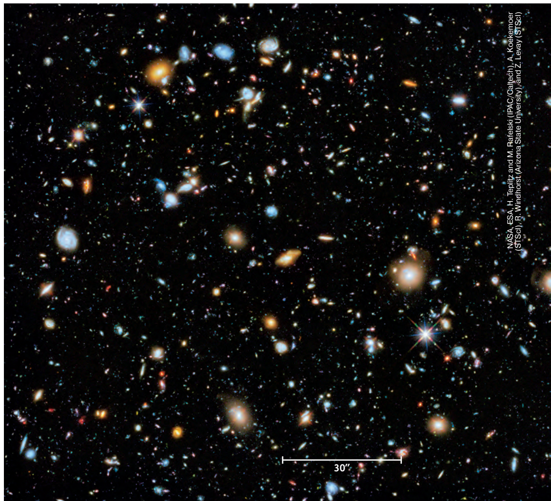
▲ Ночью на небосводе невооруженным глазом видны красивейшие россыпи звезд, поэтому ночное небо мы называем «звездным». Космический телескоп Hubble «видит» совершенно другое небо: практически все объекты, запечатленные на этом снимке — галактики. В поле зрения попала всего пара звезд Млечного Пути (их можно отличить по четырем характерным дифракционным лучам). Масштабная линейка соответствует тридцати угловым секундам, т.е. 1/60 видимого диаметра полной Луны.
