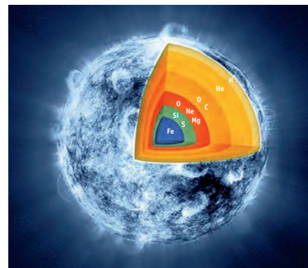
▲ Так предположительно выглядит ядро массивной звезды непосредственно перед ее взрывом как Сверхновой
